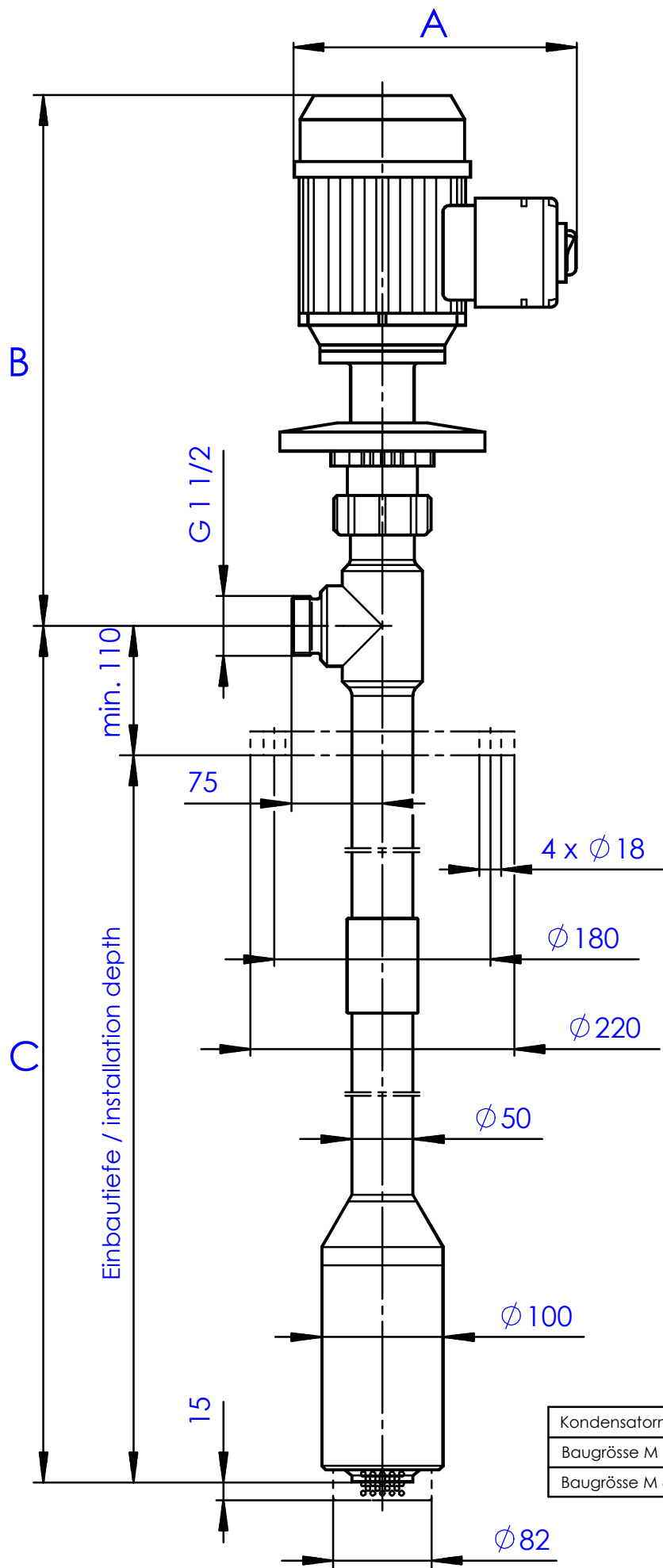
Tauchkreiselpumpe B50 Submersible centrifugal pump B50
