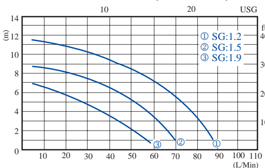
NH-250PS-F 50Hz Nominal speed 2,700 r.p.m
