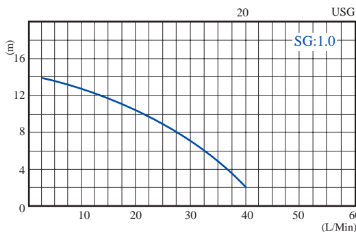
NH-200PS-F-Z 50Hz Nominal speed 2,500 r.p.m
