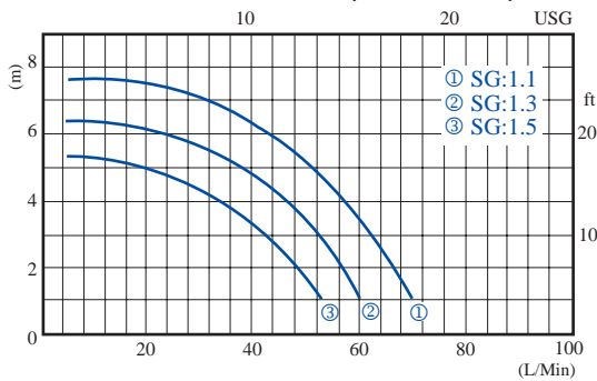
NH-200PS-F 50Hz Nominal speed 2,500 r.p.m
